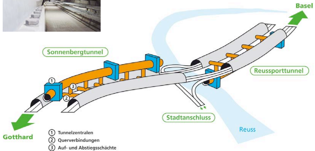
Werkleitungsstollen Reussport und Sonnenberg
