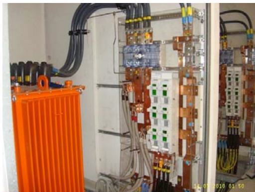
Zuleitungen aufschalten Tunnelzentrale Reussport Nord
